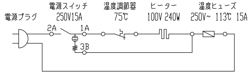
回路図
